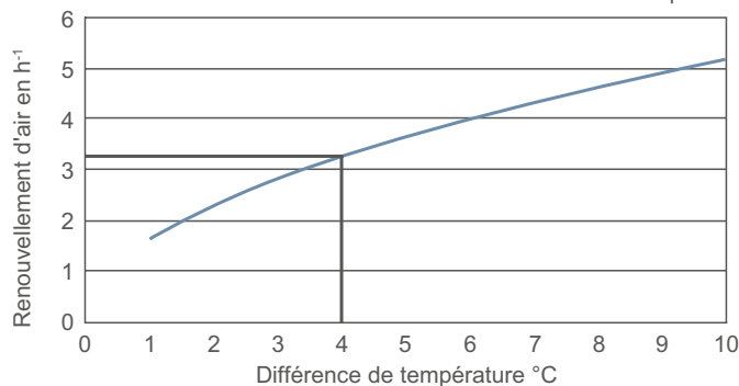
Renouvellement d'air calculé avec ascendance thermique
