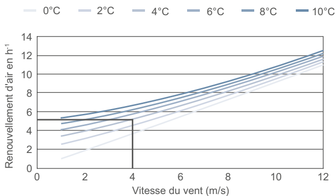
Renouvellement d'air calculé avec ascendance thermique et vent
